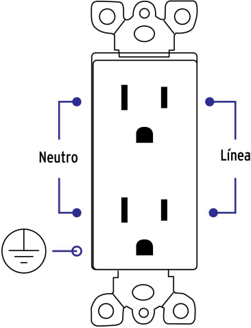
Diagrama de conexión
