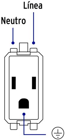
Diagrama de conexión
