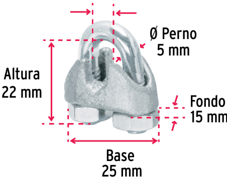
Diámetro del cable 3/16" (5 mm)
