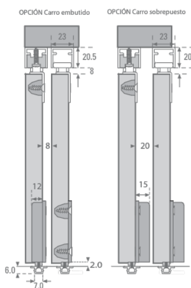
Vista Lateral
